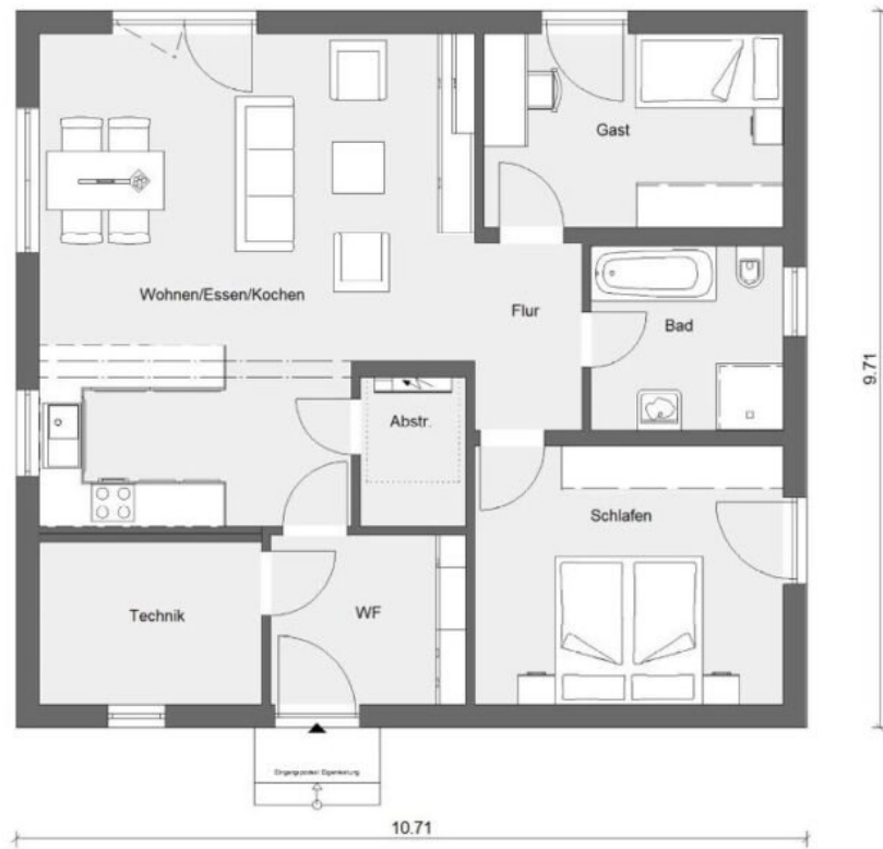
Plan E 10-087.7 · Erdgeschoss · Nettogrundfläche 86,52 m 2 · Wohnfläche 79,75 m 2
